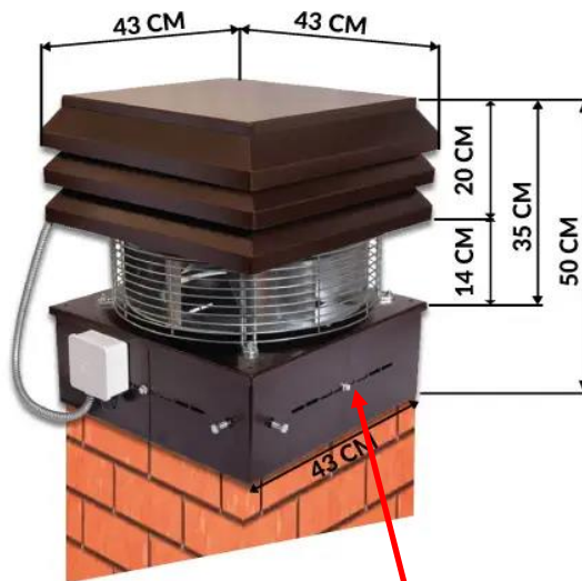
BASE REGISTRABILE
